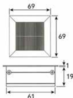
Passage de câbles sans couvercle type NC - double brosse noir
